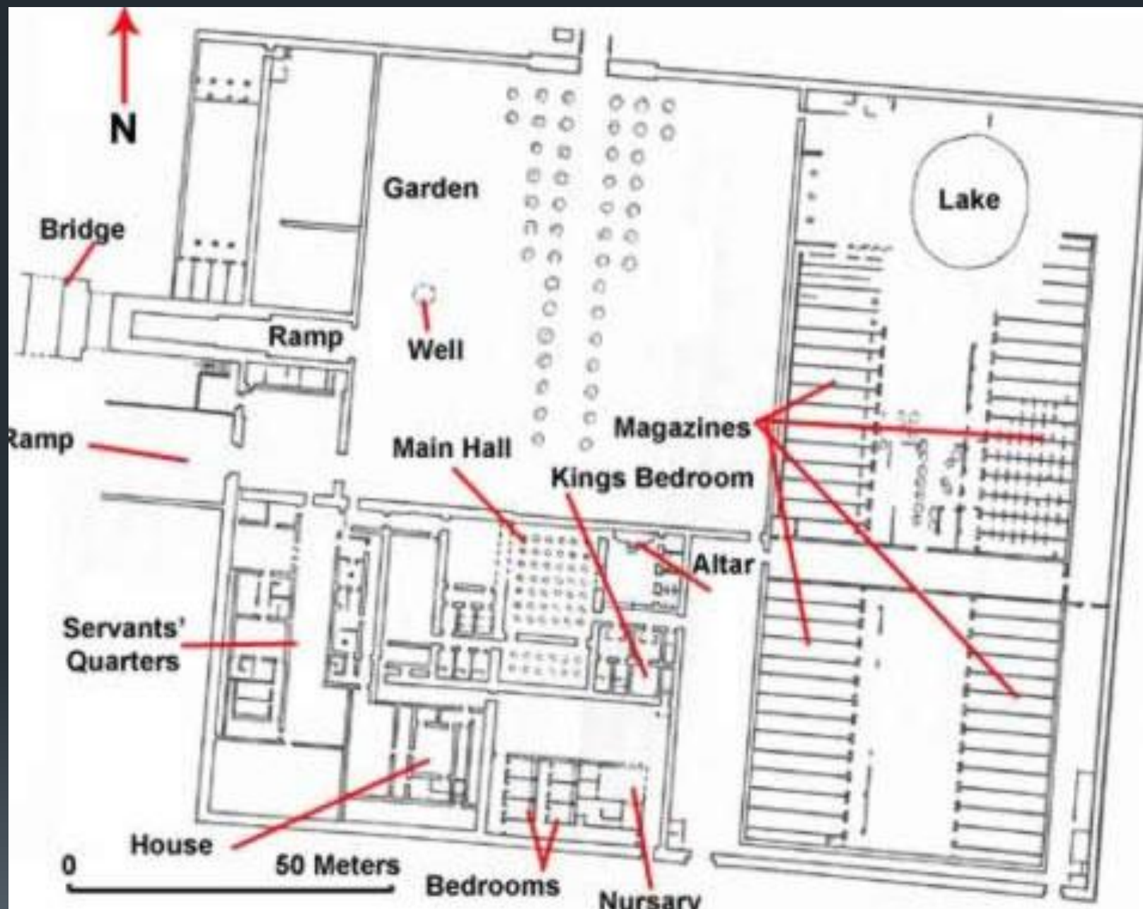
královský palác „the king's house“ v Amarně, Nová říše
